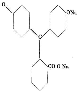
Chinoides Salz.
